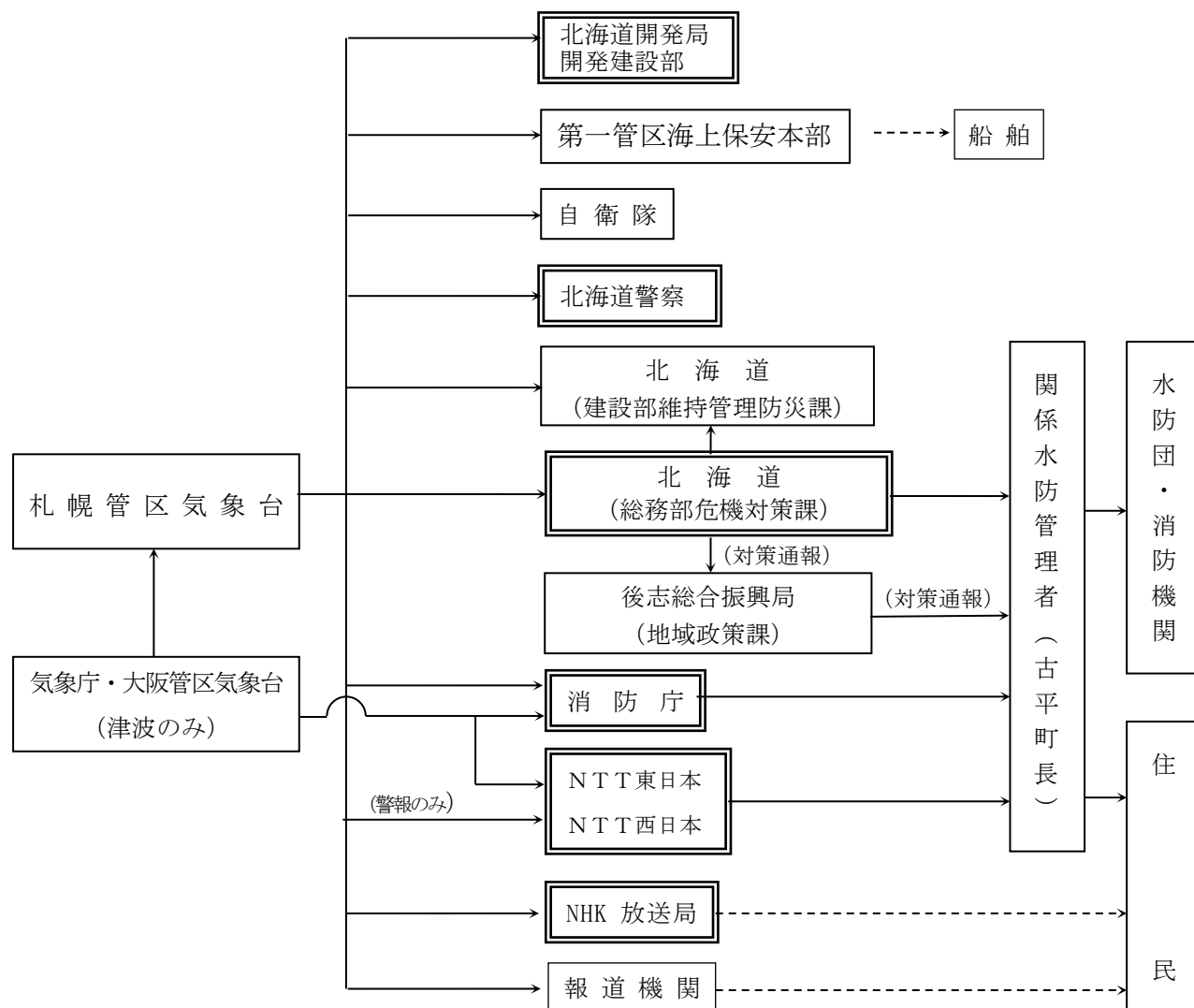
圖表 水防活動用氣象等警報・氣象注意報傳達系統圖
