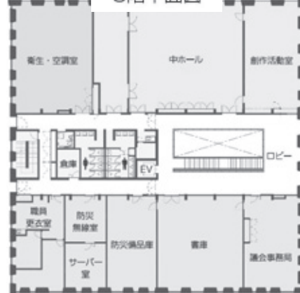
3階平面図
