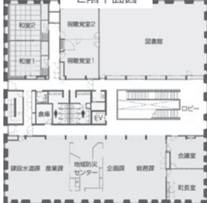
2階平面図
