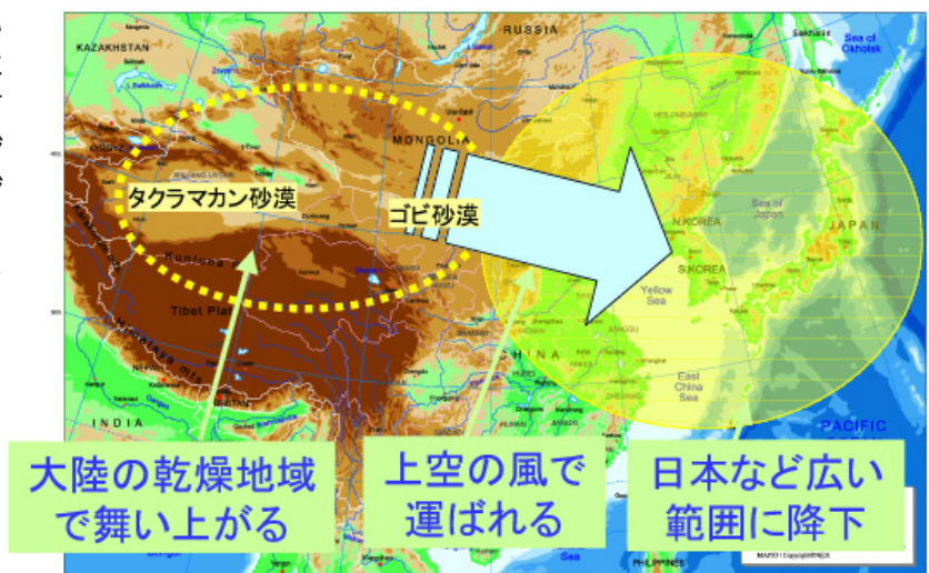
黄砂の発生と飛来
